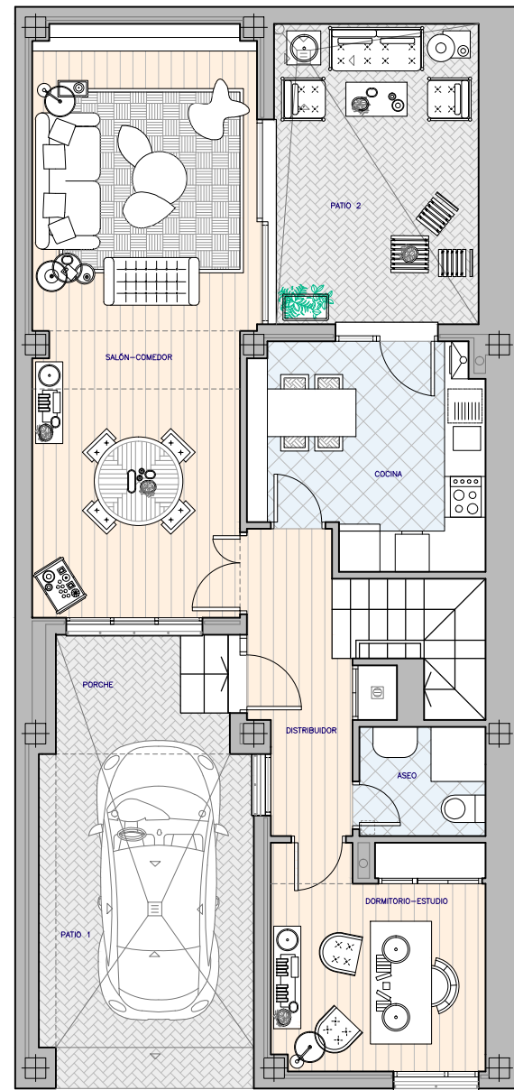
PLANTA BAJA
